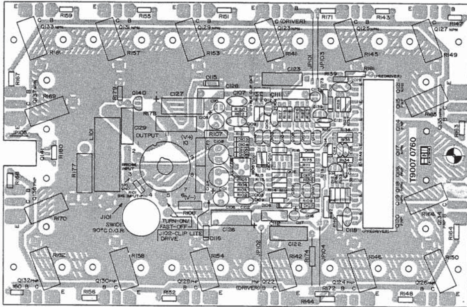
TOP SIDE
