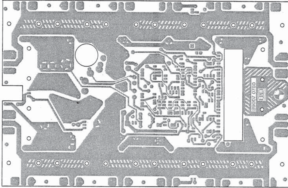
BOTTOM SIDE
