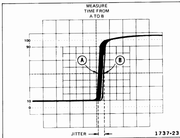
Fig. 25. Pulse jitter.
