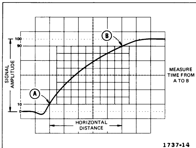
Fig. 21. Risetime.
