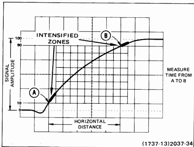
Fig. 34. Risetime.
