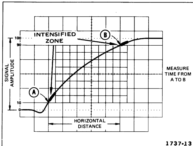
Fig. 30. Risetime.
