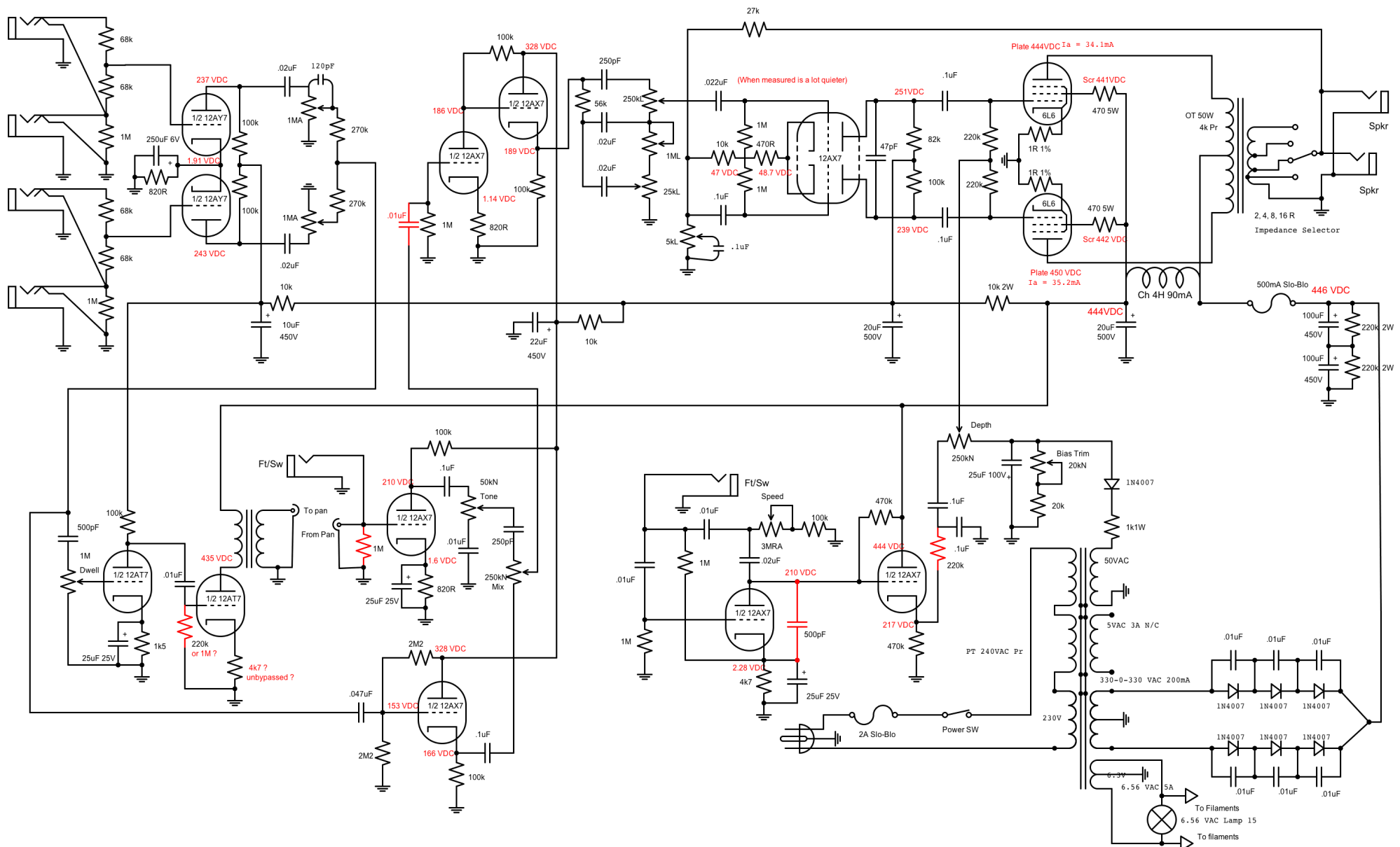
Tweed Bassman + 6G15/BF Reverb 6G16 Trem tubeswell Rev 12 e 8/04/09 Page #
