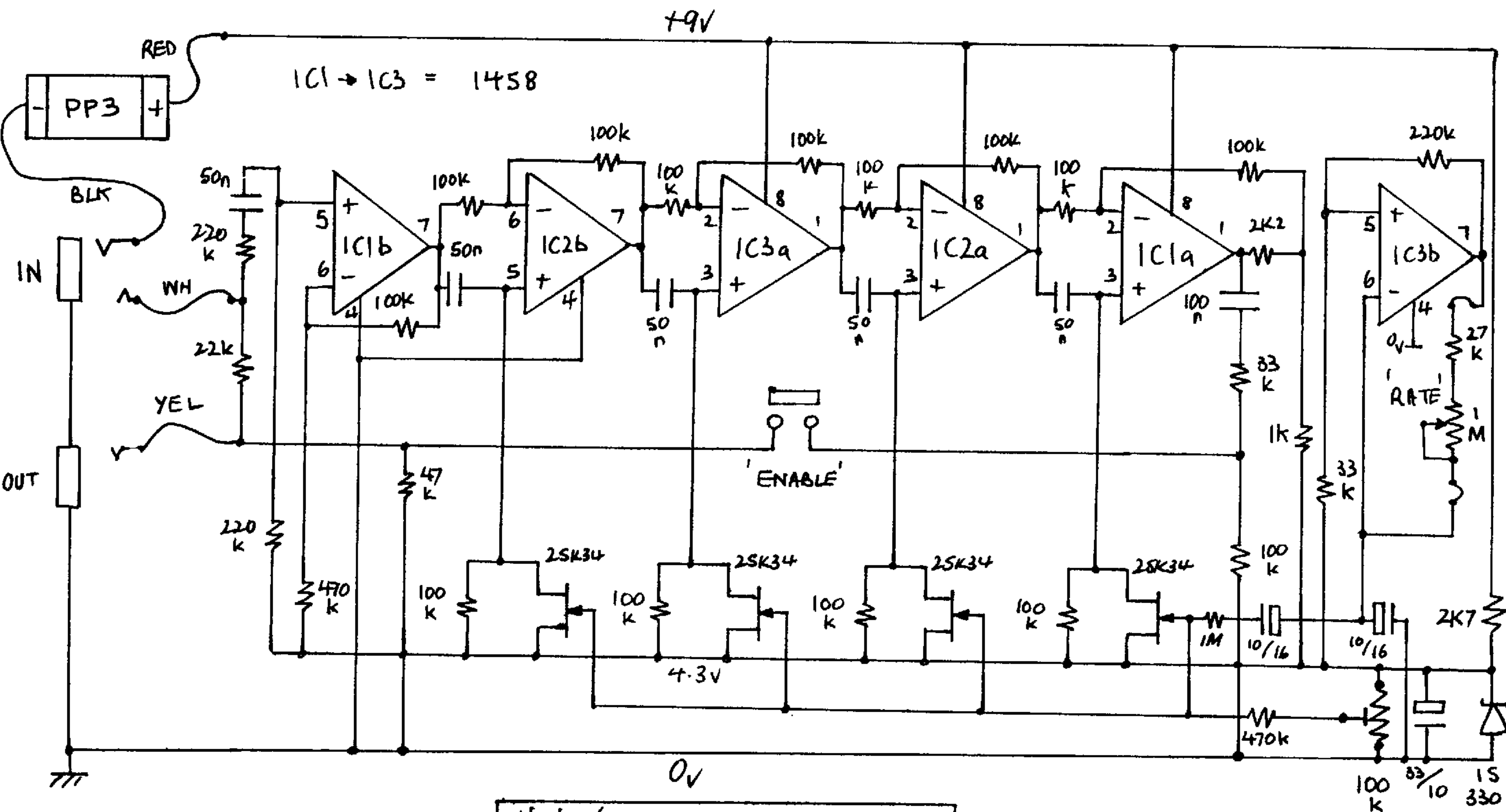
UNIVOX MICRO FAZER
