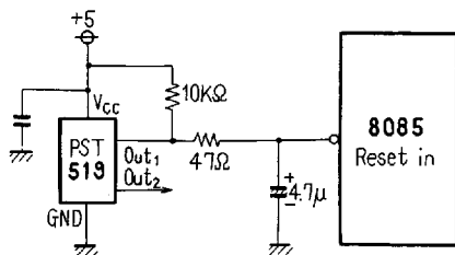
[Fig. 3] 8085 の Reset 回路/Reset circuit of 8085
