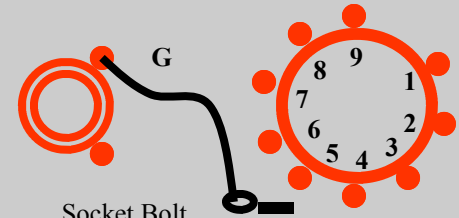
12AX7B
